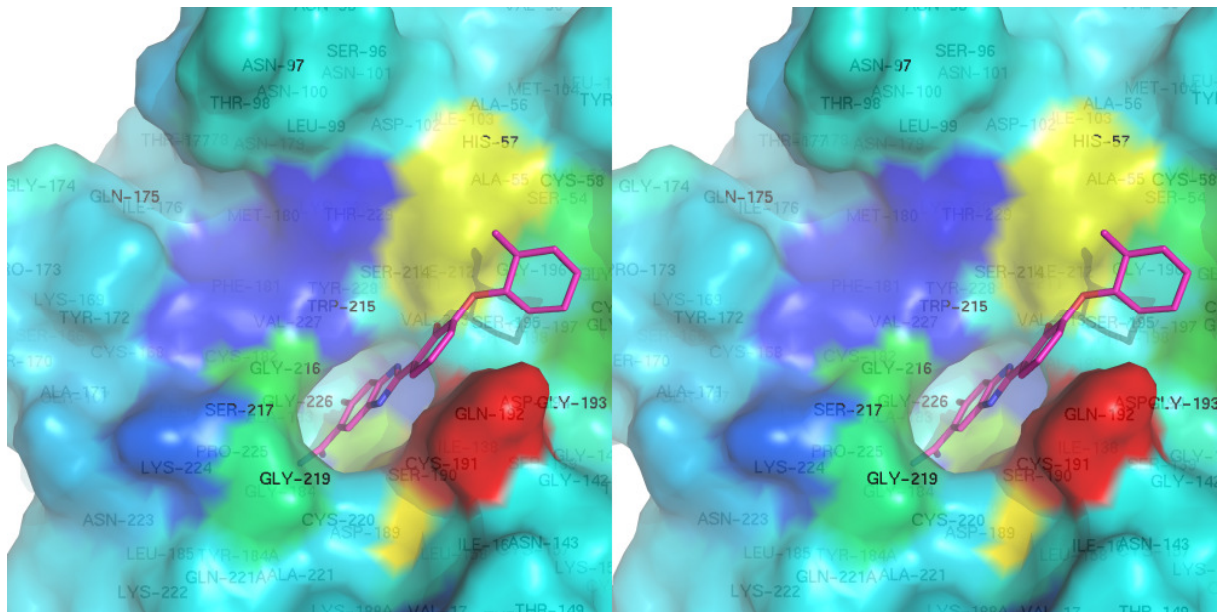
B_trypsin-diff-vdw-coeff_try-thr.png
